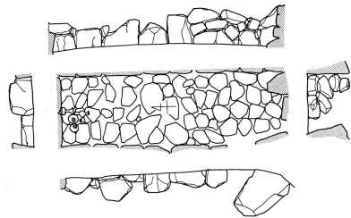
第25図 石室奥面図(第6号古墳)
