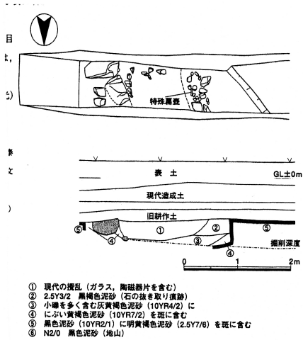
図36 4号墳石室平面図・断面図 (1:50)
