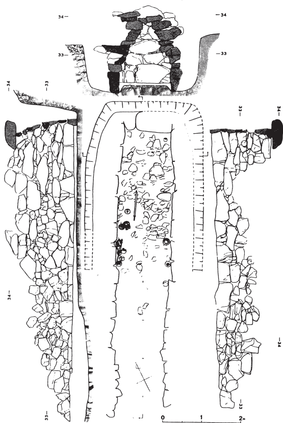
第7图 1号墳第2主体部实测图 1/100
