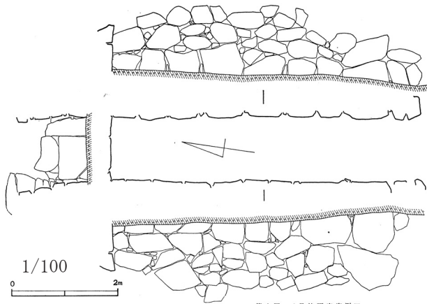
第3図 1号墳石室実測図
