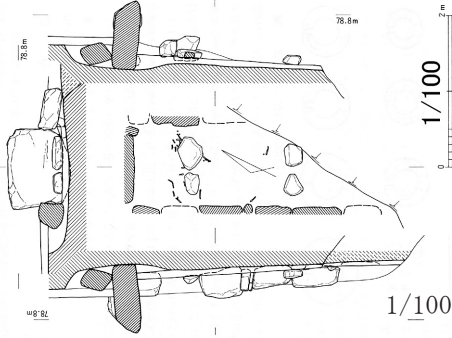
1/100 1/100 図64 ST-6 石室平・断面図
