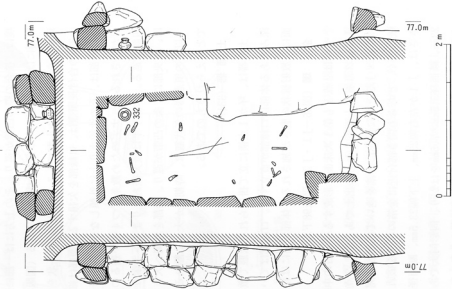
1/100 図57 ST-5 石室平・断面図
