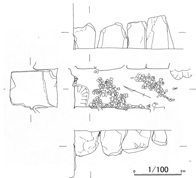
fig. 25 石室平面・立面図
