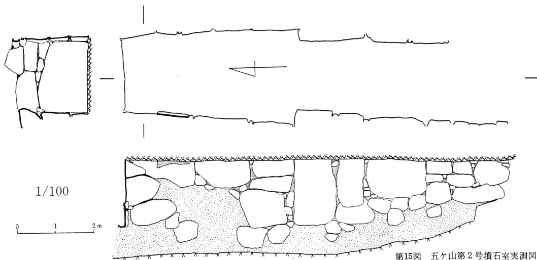
第15図 五ヶ山第2号墳石室実測図
