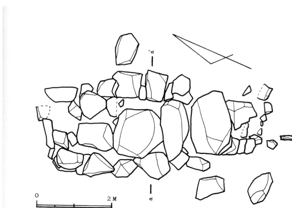
(1) 中筋山手古墳群 7号墳 石室実測図
