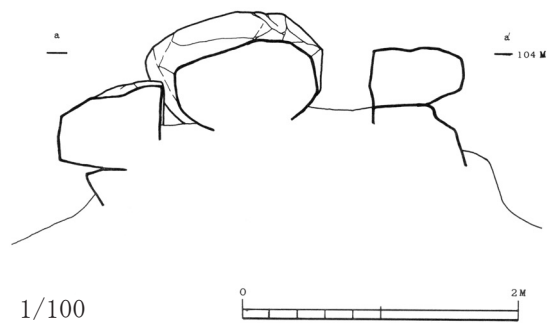
(2) 中筋山手古墳群 7号墳 石室断面図
