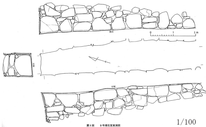
第8図 9号墳石室実測図
