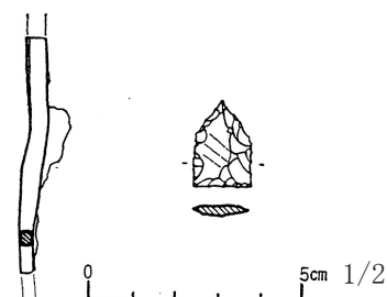
第15図 10号墳遺物実測図
