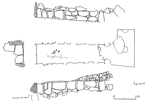
图 64 雲雀山東尾根古墳群A群5号墳石室 1/100
