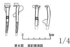
第9図 鉄釘実測図
