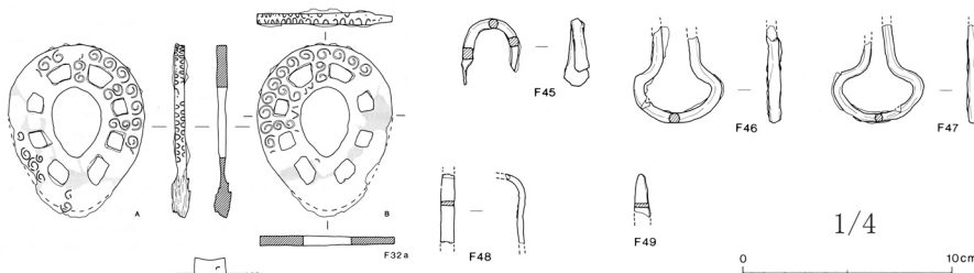
挿図47 2号墳鉄器(4)
