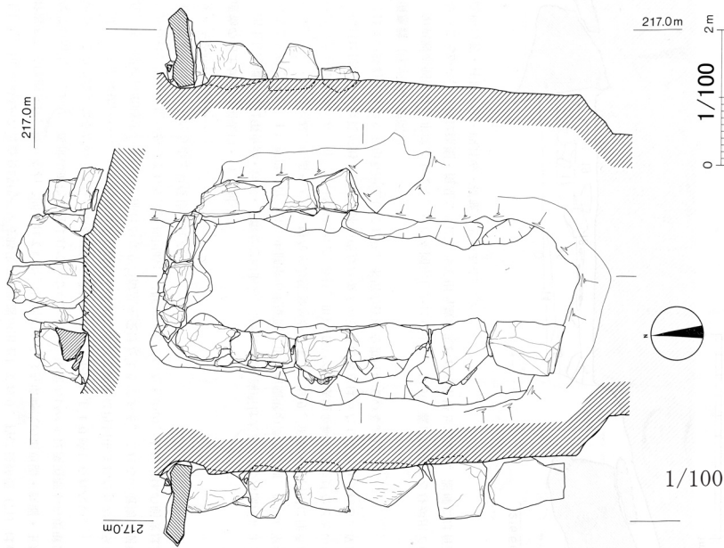
挿図40 2号墳石基測量図
