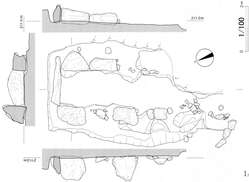
插图21 1号墳石室平面図
