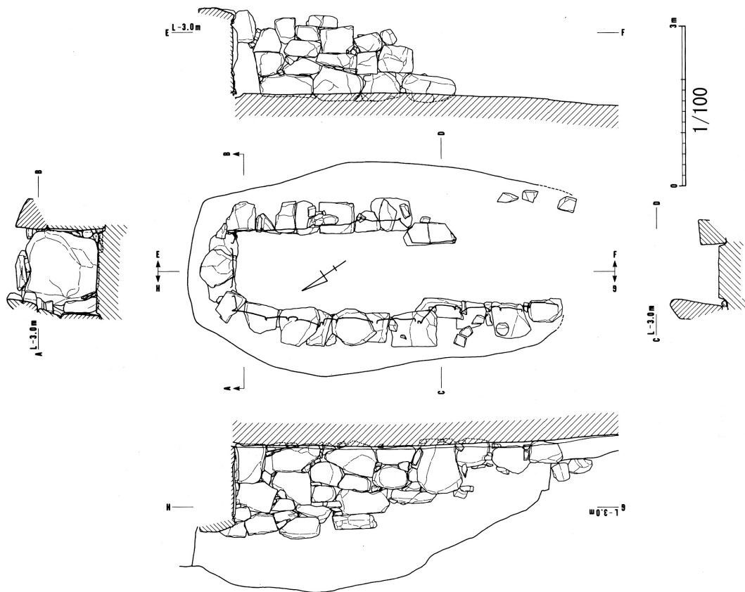
第50図 石室実測図
