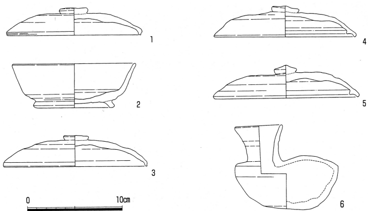
第8図 村東山古墳遺物実測図
