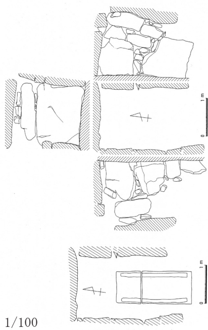
第6図 石室実測図
