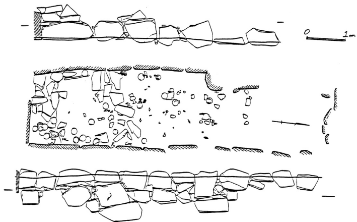
第2図 横穴式石室実測図 (A区)
