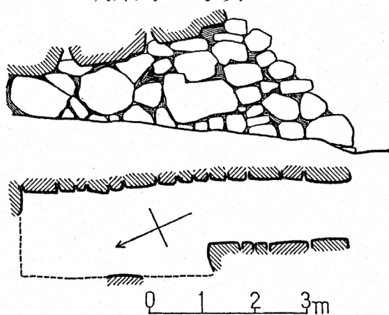
図2-36 明楽寺3号墳横穴式石室実測図
