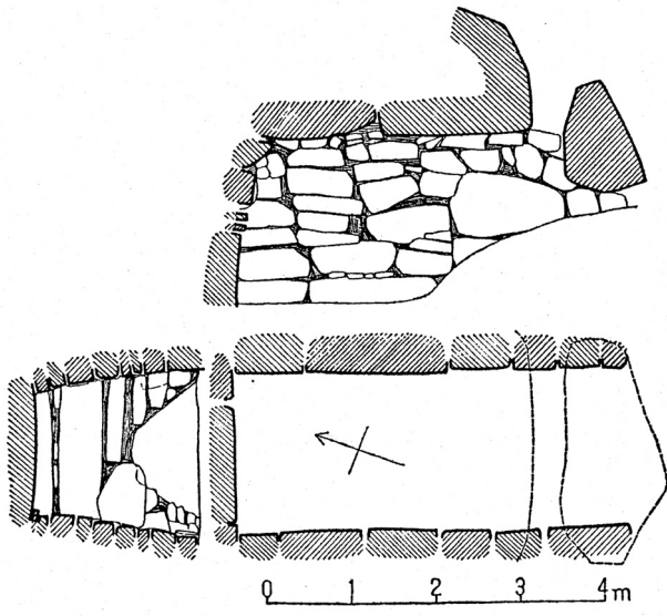
图 2-31 谷古墳横穴式石室実測図
