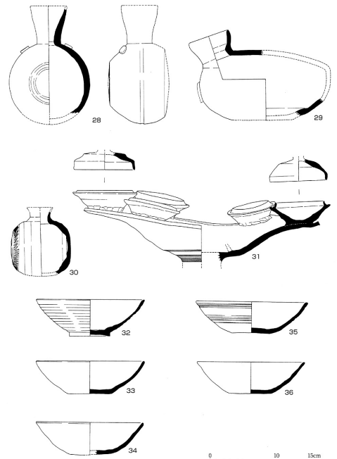
第35図 26号墳出土遺物実測図 2 1/8
