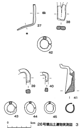
26号墳出土遺物実測図 3
