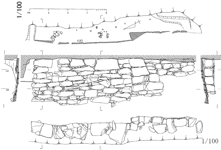
第33図 26号墳横穴式石室実測図
