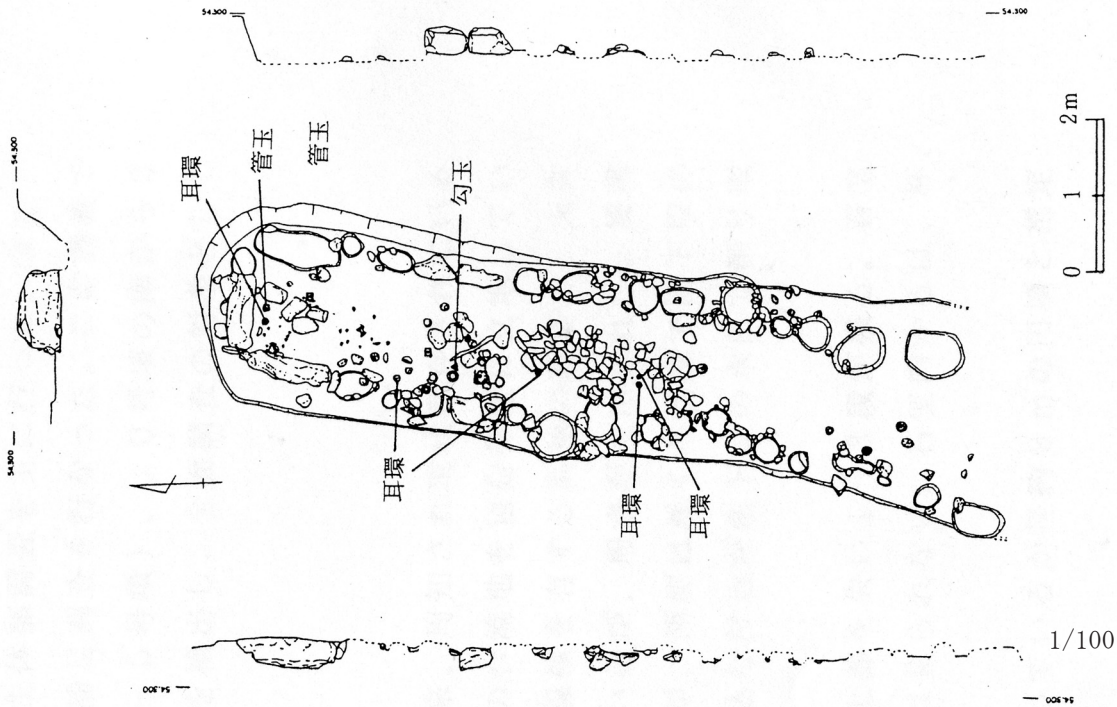
主体部平面図 1/100
