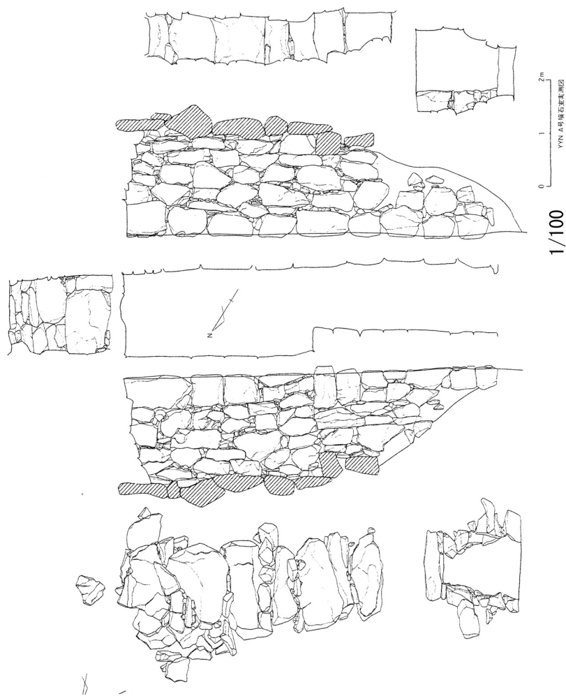
図12 吉馬滑A号墳実測図
