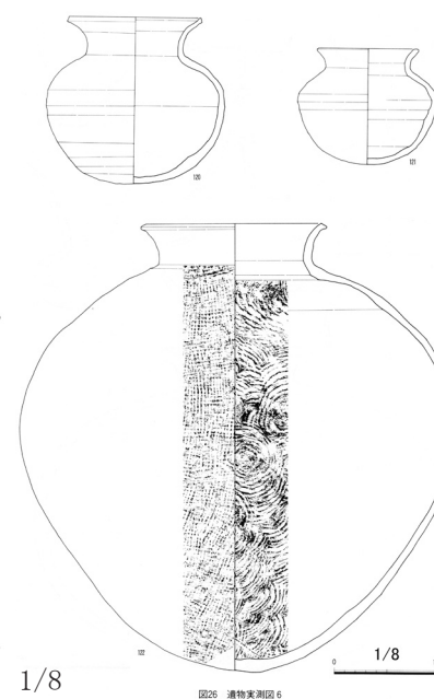
图26 遗物实测图6
