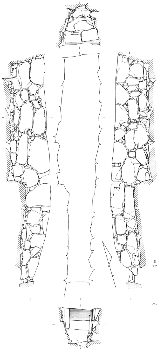
图 42 山崎大塚古墳石室実測図
