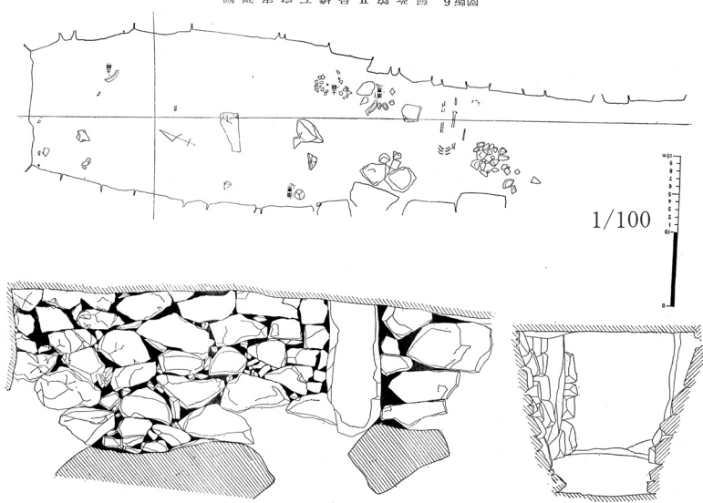
図版6 阿弥陀II号墳石室実測図
