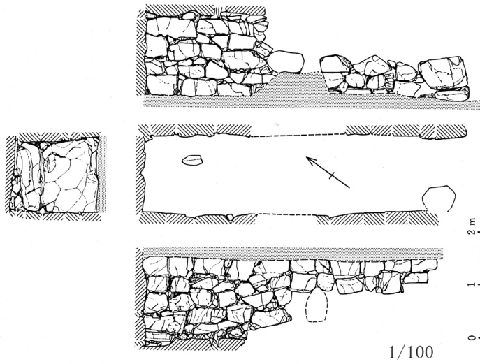
図 159 中山2号墳 石室実測図
