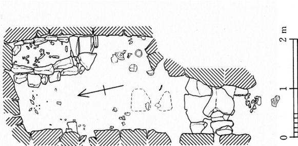
図 157 中山3号墳 石室実測図
