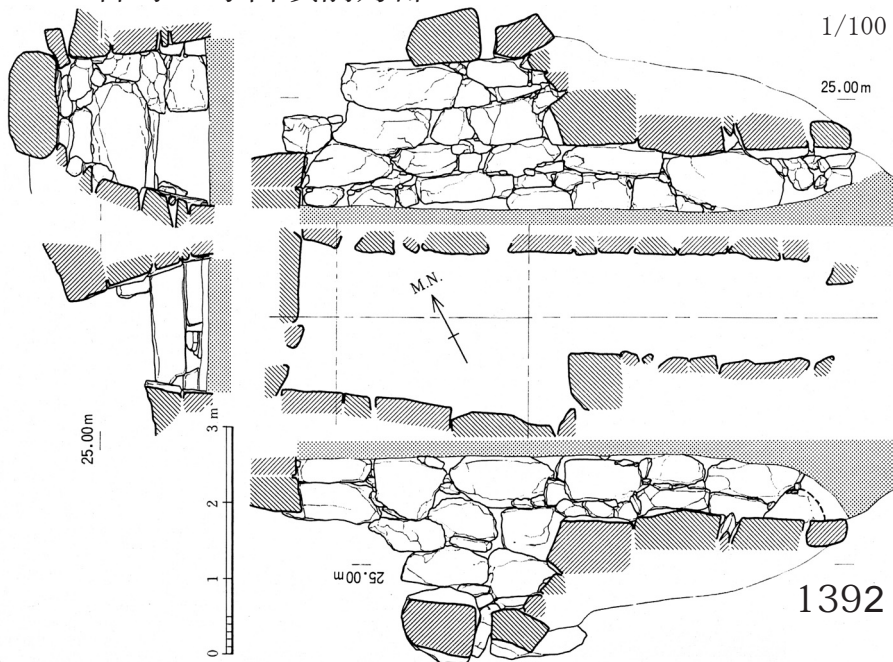
図 135 二塚2号墳 石室実測図
