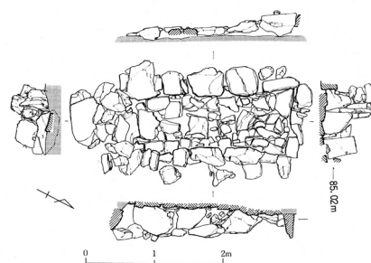
図 164 カメ焼谷3号墳 石室実測図
