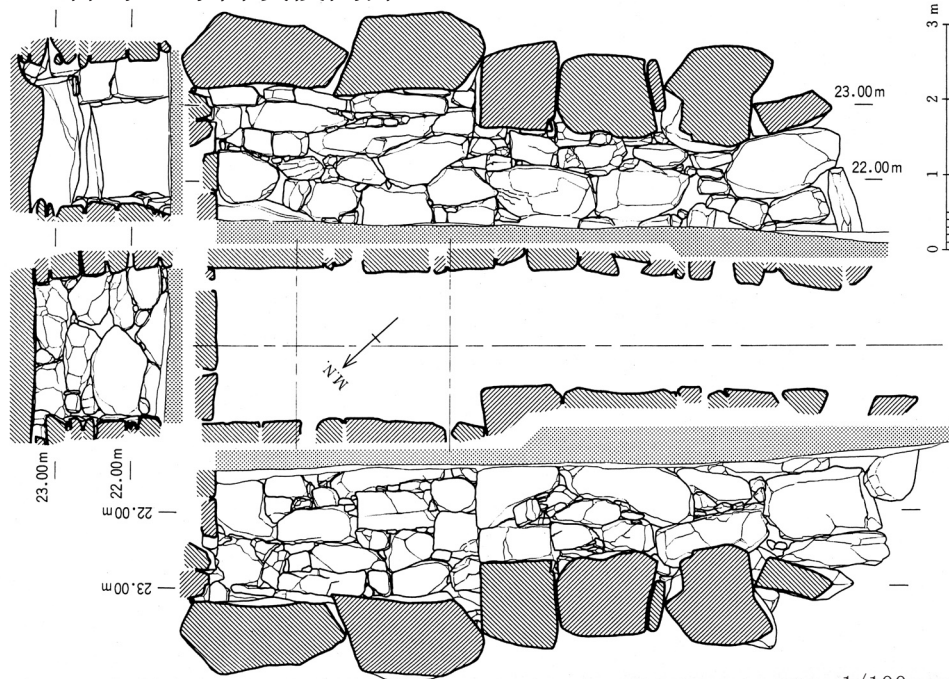
図 134 二塚1号墳 石室実測図
