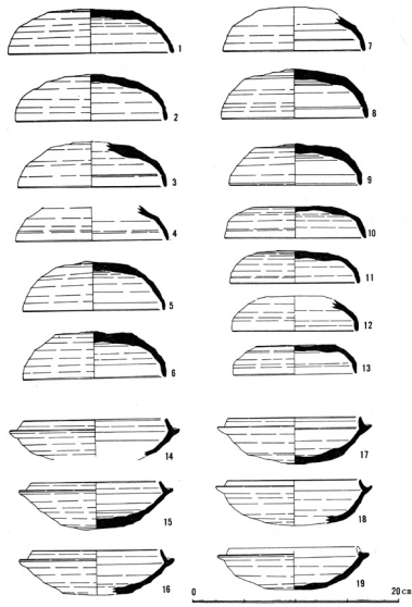
第8回 二子塚古墳出土須恵器実測図
