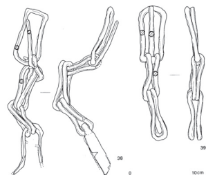
第79図 龍子向イ山1号墳出土鉄器実測図(3) [馬具]
