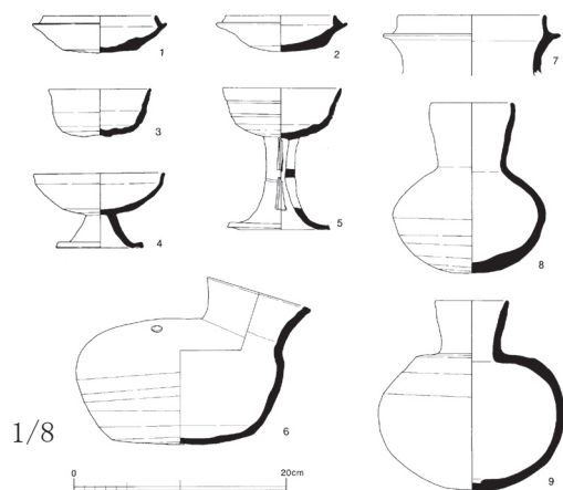
第91図 龍子向イ山2号墳出土土器実測図
