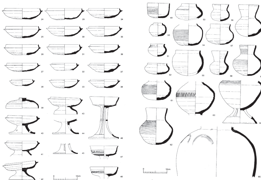
第70図 龍子向イ山1号墳出土須恵器実測図(2) 1/8
