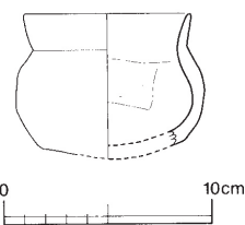
第102図 土師器実測図 1/4
