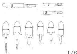
第104図 龍子向イ山3号墳鉄器実測図(2)
