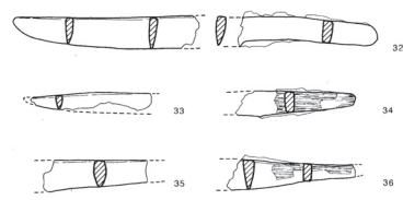
第77図 龍子向イ山1号墳出土鉄器実測図(2) [刀子]
