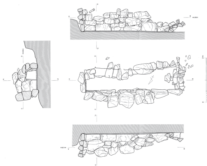
第109図 龍子向イ山4号墳石室 実測図
