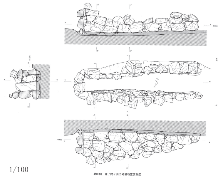
第88図 龍子向イ山2号墳石室実測図
