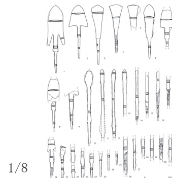
第78図 龍子向イ山1号墳出土鉄器実測図(1) [鍬頭]
