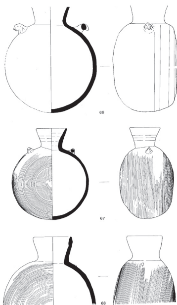
第72図 龍子向イ山1号墳出土須恵器実測図(4)
