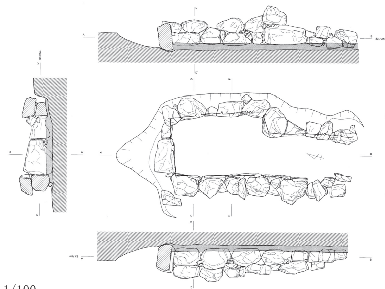
第99図 龍子向イ山3号墳石室実測図
