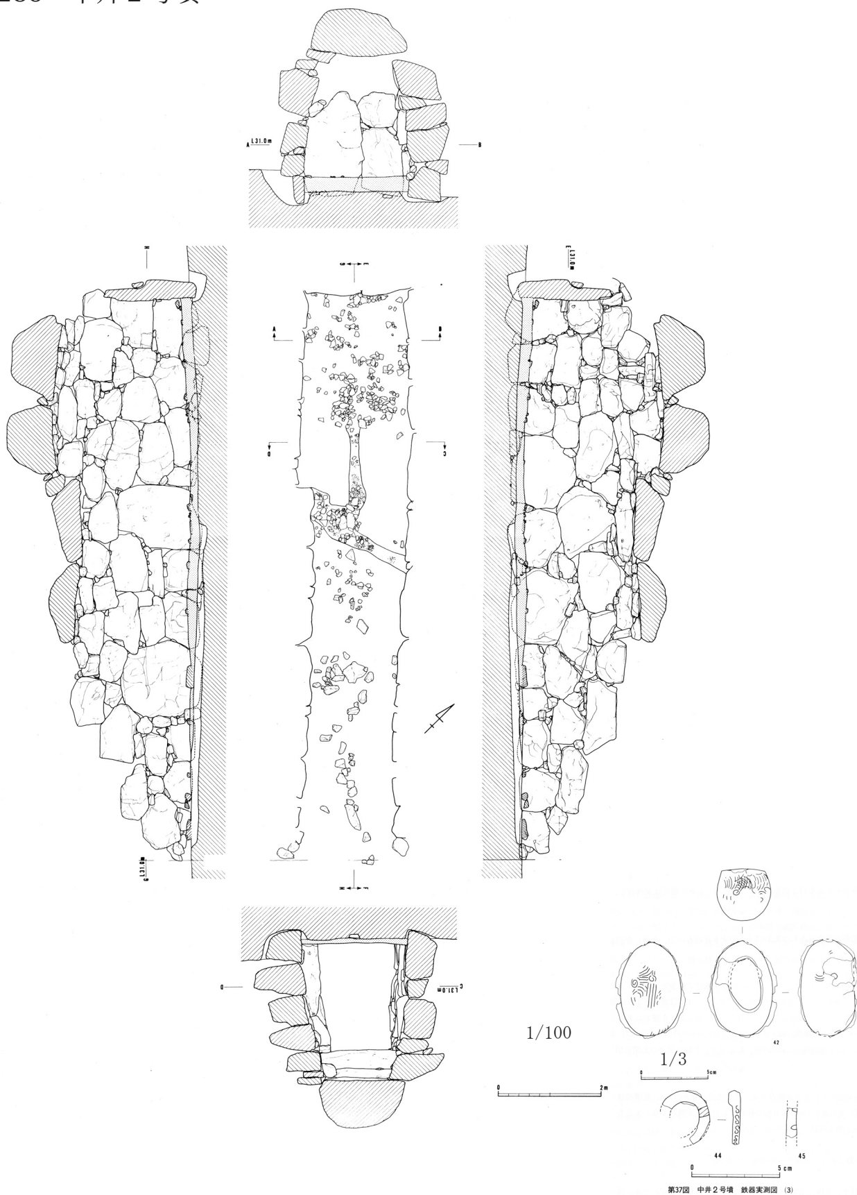
第37図 中井2号墳 鉄器実測図 (3)
