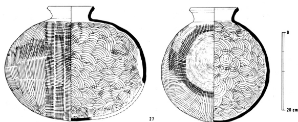
第19図 中井1号墳須恵器実測図 (2)
