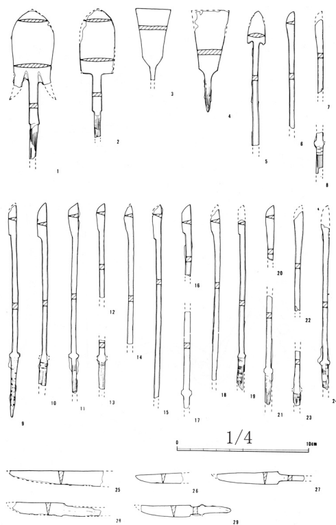
第35図 中井2号墳 鉄器実測図(1)
