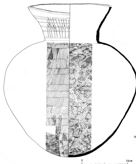
第33図 中井2号墳 須恵器実測図(2)
