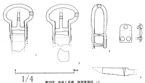
第20図 中井1号墳 鉄器実測図 (1)
