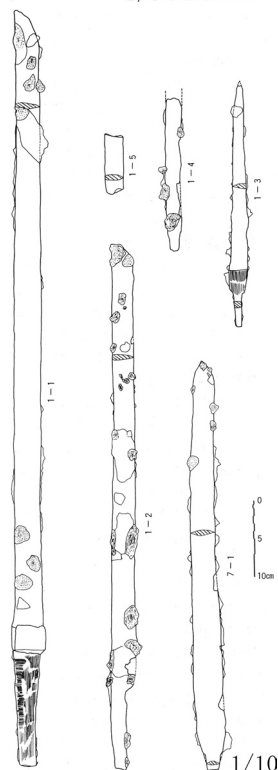
図96 1号墳鉄刀 (1-5)、7号墳鉄剣
