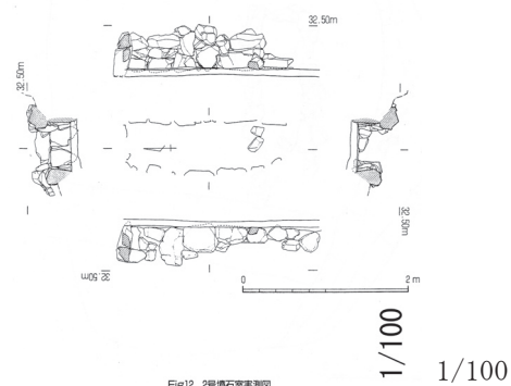
Fig.12 2号墳石室実測図
