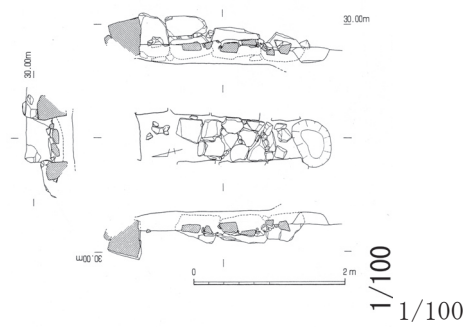
Fig.9 1号墳石室実測図
