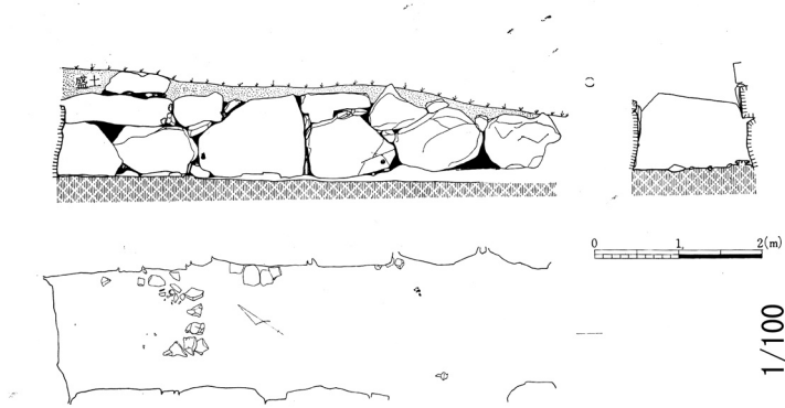
第11図 第1号古墳石室実測図
