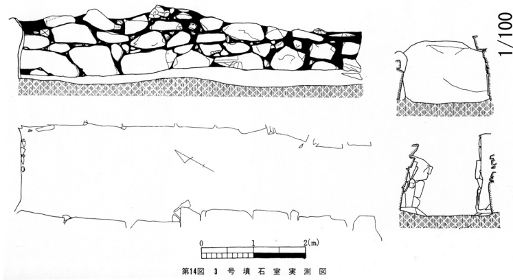
第14図 3号墳石室実測図
