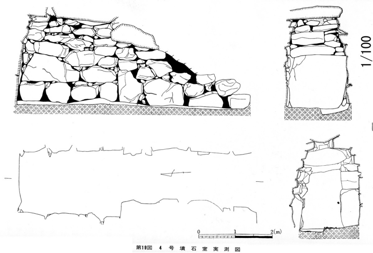
第19図 4号墳石室実測図
