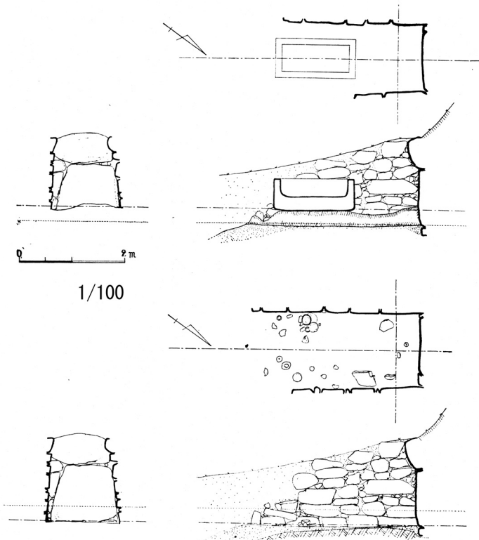
第54図 ヒシノタイ古墳石室美測図
