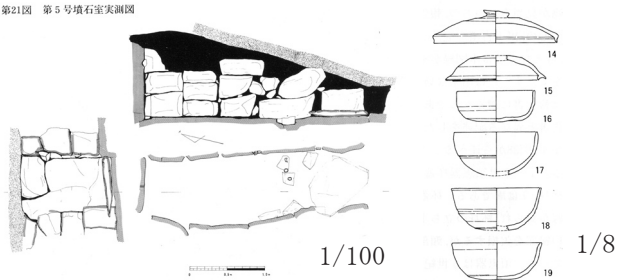
第21図 第5号墳石室実測図
