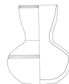
第45図 第9号墳出土遺物実測図Ⅲ
