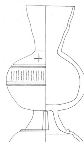
第48図 第9号墳出土遺物実測図Ⅵ
