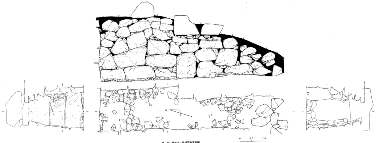
第7図 緑ヶ丘2号墳石室実測図
