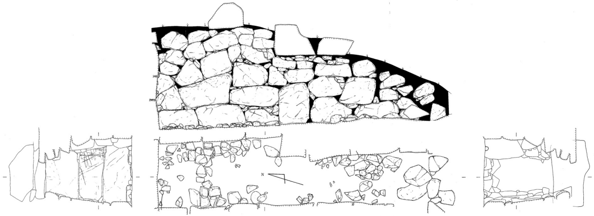
第7図 緑ヶ丘2号墳石室実測図
