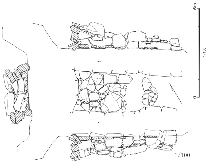
fig. 45 石室実測図
