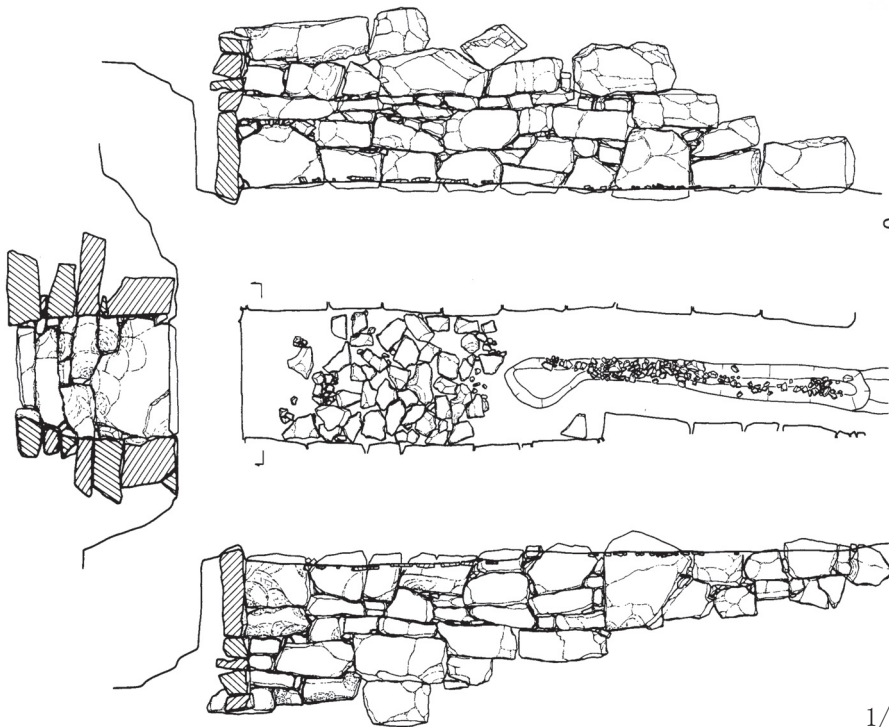
fig. 100 石室実測
