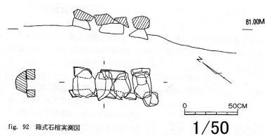
fig. 92 葬式石棺実測図
