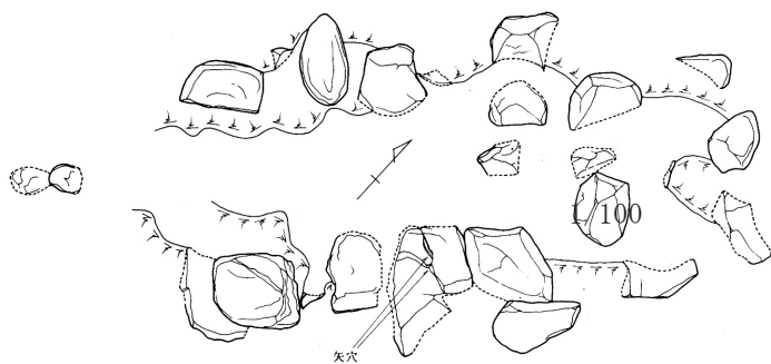
第37図 毘沙門4号墳石室上面実測図
