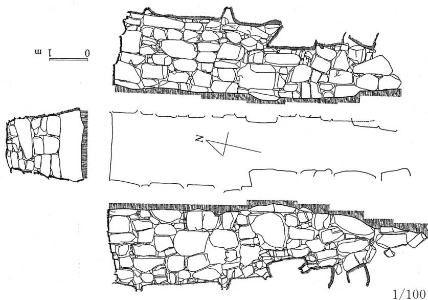
第13図 曲田山古墳石室実測図
