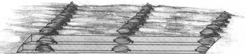
図 20 最初の堤体の築造方法
