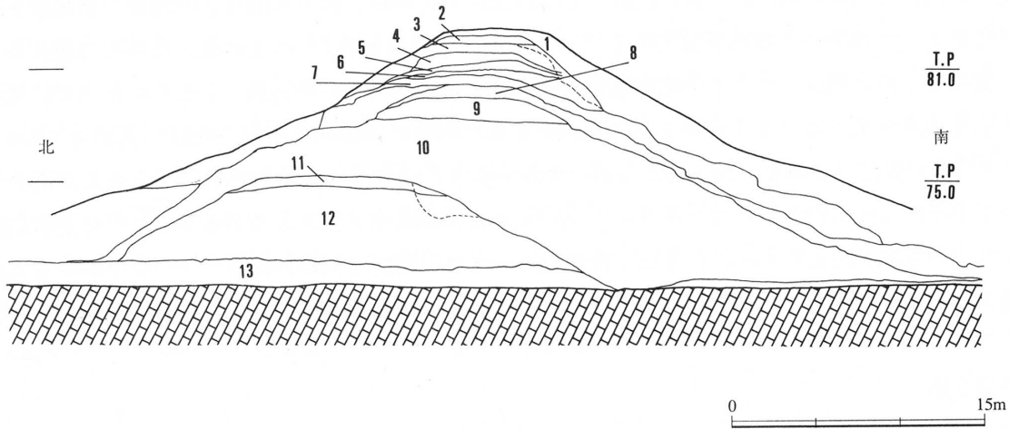
图6 北堤断面图 (中樋地点东侧) (S=1/400)
