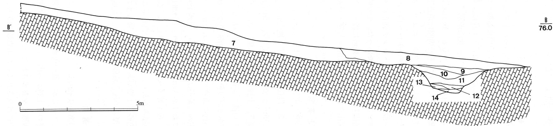
図 230 狭山池 4 号窯灰原土層断面図 (1/80 · 1/100)
