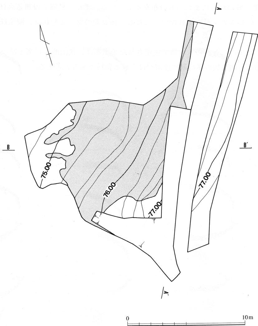
图 231 狭山池 4 号灰原平面图
