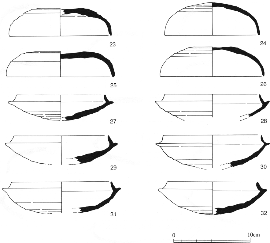
图 197 狭山池 2 号窑灰原出土遗物 (2) (23~32: 中層灰原)
