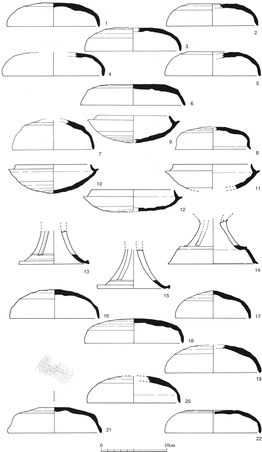
图 196 狭山池 2 号熏灰原出土遺物 (1) (1~14: 上層灰原、15~22: 中層灰原)
