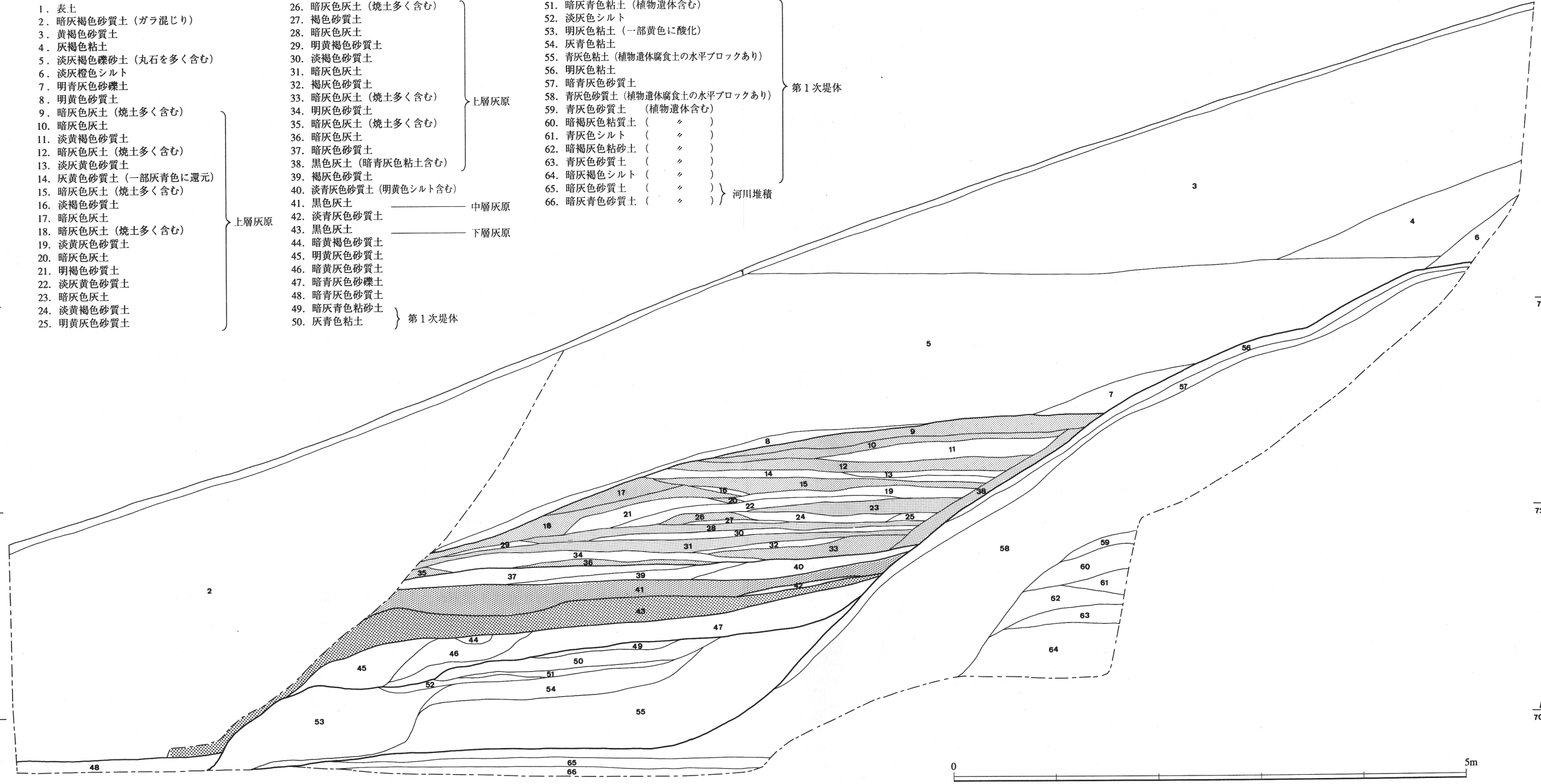
図 154 狭山池 1 号窯灰原土層断面図 (S=1/40)
