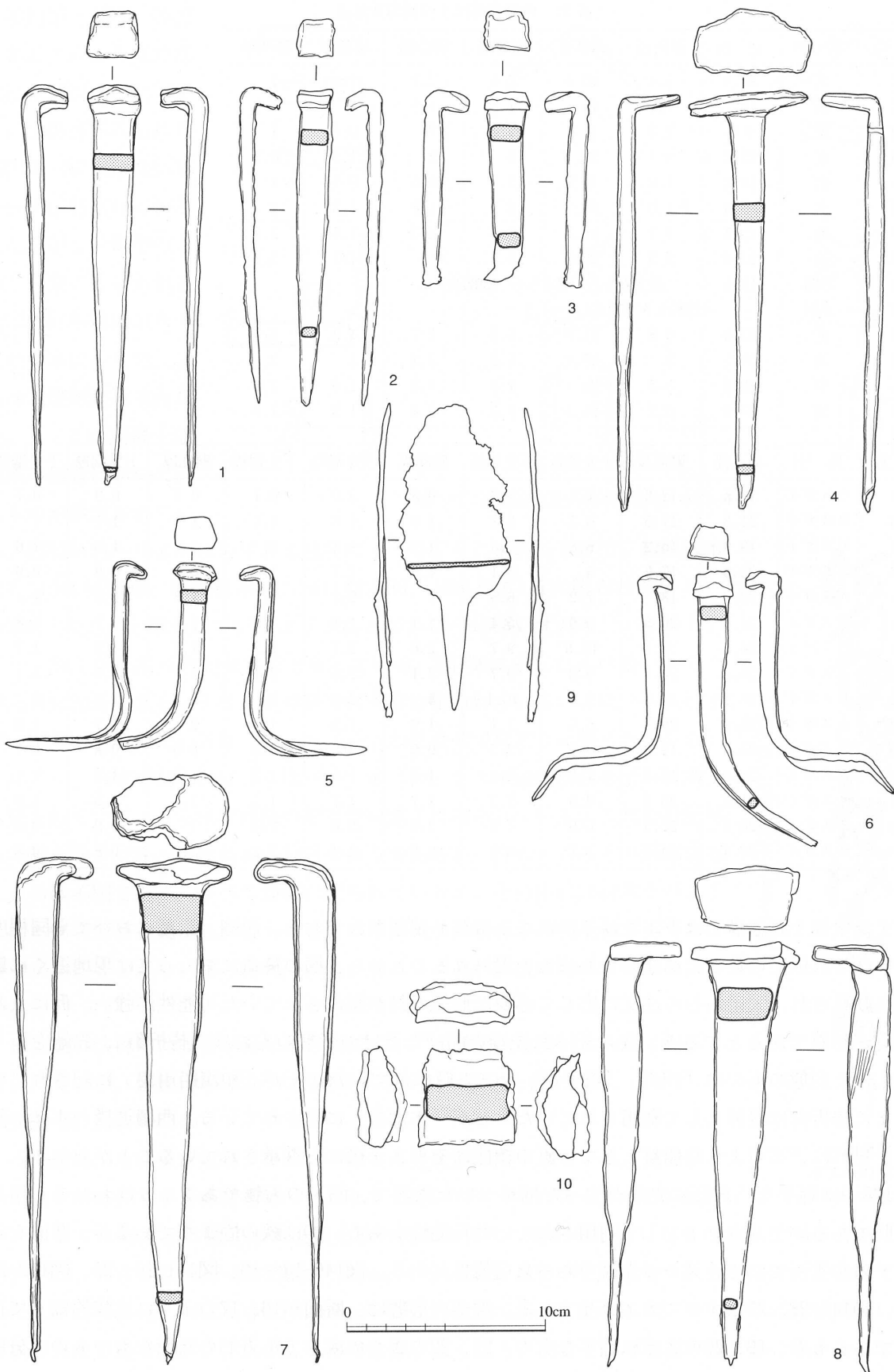
图 138 西槿遺構出土金属器实测图 (1) (S=1/3)
