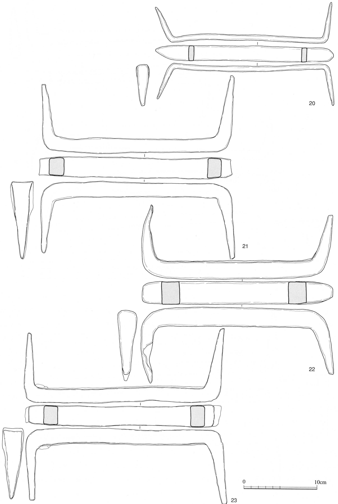
图 141 西樋遺構出土金属器实测图 (4) (S=1/3)
