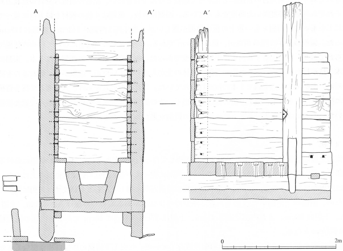
図 63 東樋上層遺構取水部断面見通し図 (記号は図60に対応) (S=1/40)
