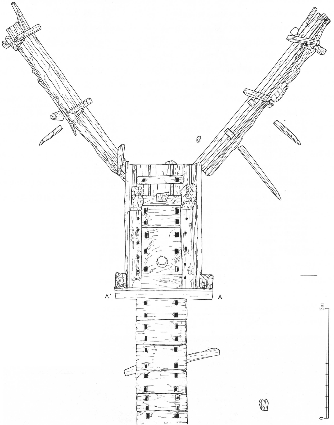
图 60 東樋上層遺構取水部平面図 (S=1/40)
