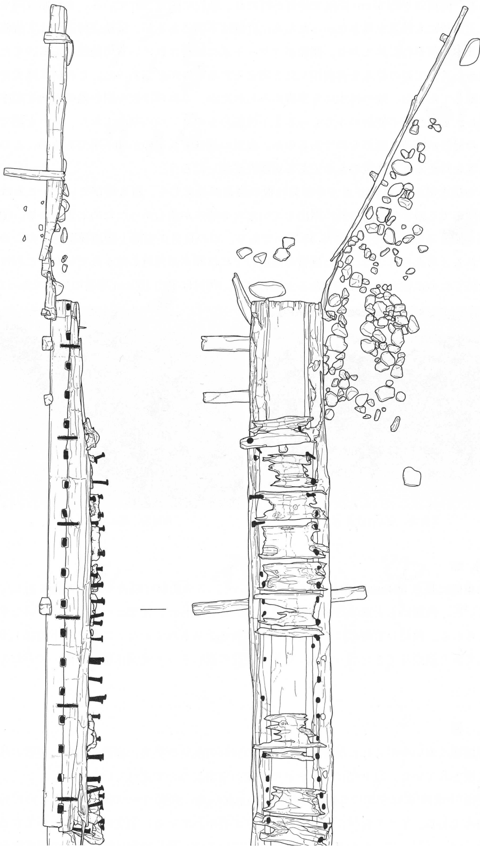
图 64 東樋上層遺構排水部平立面图 (S=1/40)
