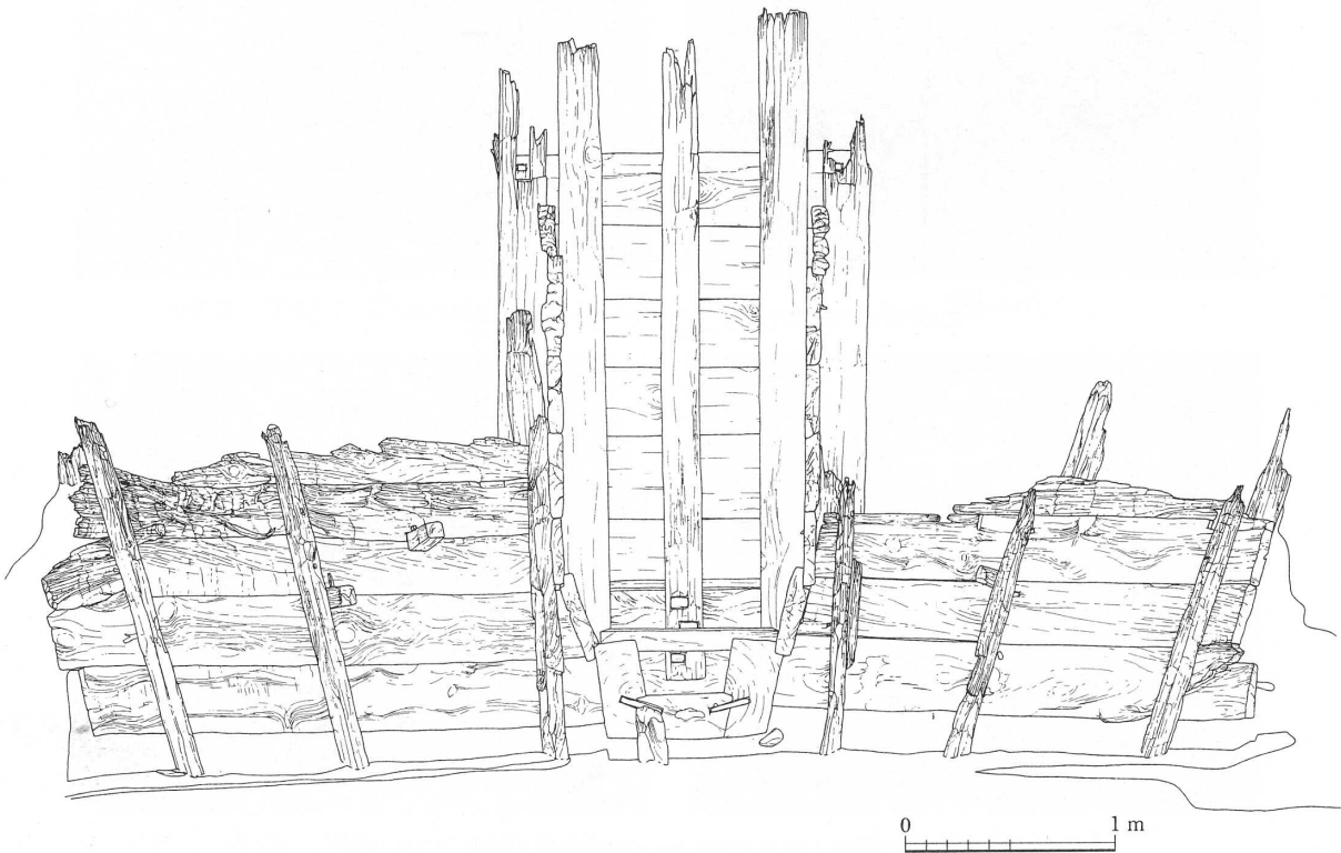
図 61 東樋上層遺構取水部立面図 (南から) (S=1/40)
