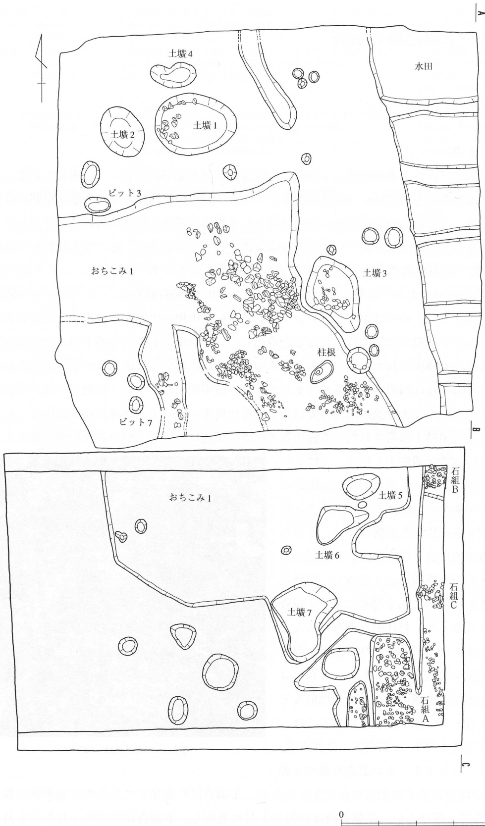
図 254 池尻遺跡 (I) A 調査区・D 調査区遺構平面図 (S=1/100)
