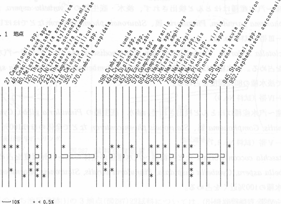
図 288 池尻遺跡(1)No.1 地点の珪藻ダイアグラム
