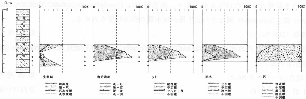
図 289 池尻遺跡(1)No. 1 地点の珪藻総合ダイアグラム
