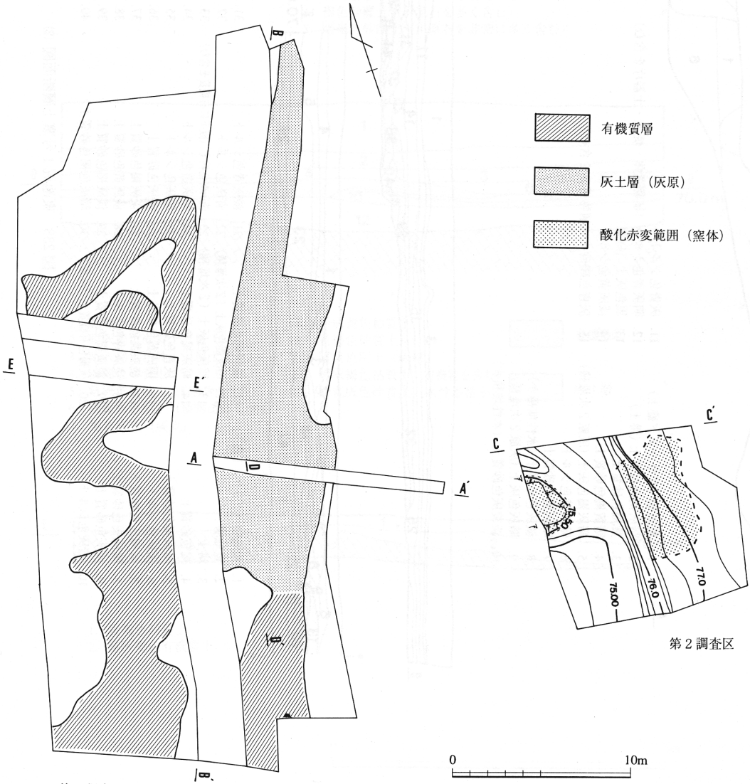
図 237 東池尻 1 号窯平面図
