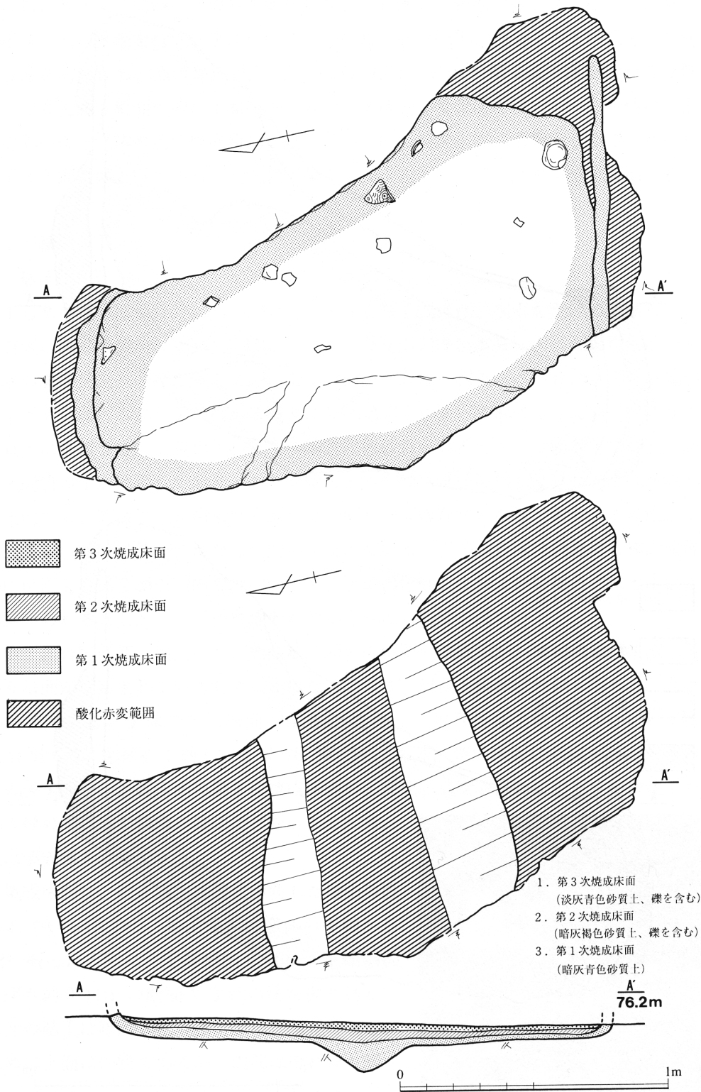
图 236 東池尻 1 号窯焼成部平面图 (2) · 土层断面图 (1)
