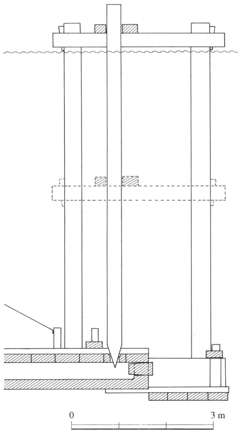
図 320 東樋下層遺構（奈良時代）取水部復元図（全体）
