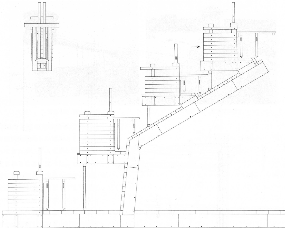
图327 西槌復元图 (S=1/150)
