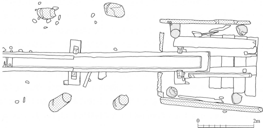
図 319 東樋下層遺構取水部 (細かいトーン；上部構造・粗いトーン；土留・トーンなし；下部構造)
