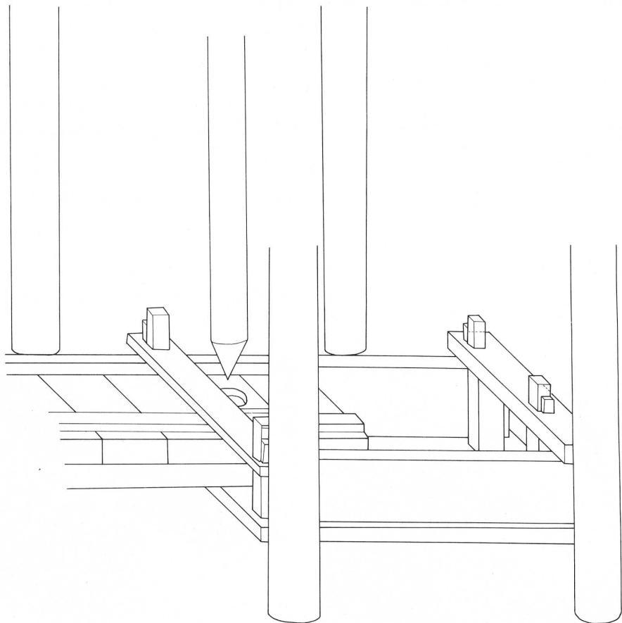
图 321 東榎下層遺構（奈良時代）取水部復元図（部分）
