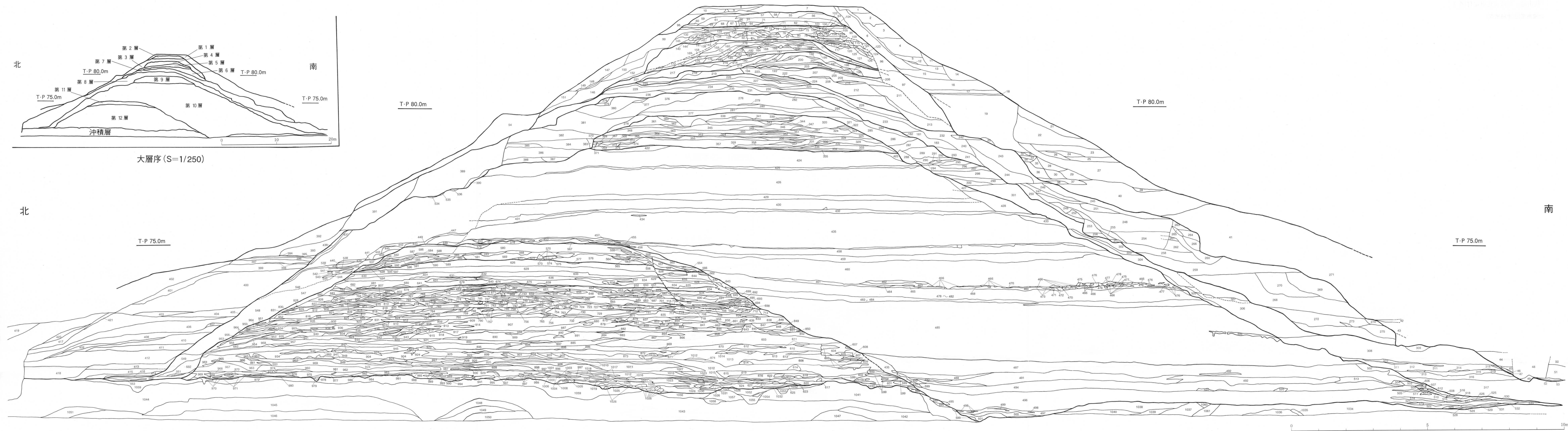
付图1 北堤断面图 (中桶地点) (S=1/50)
