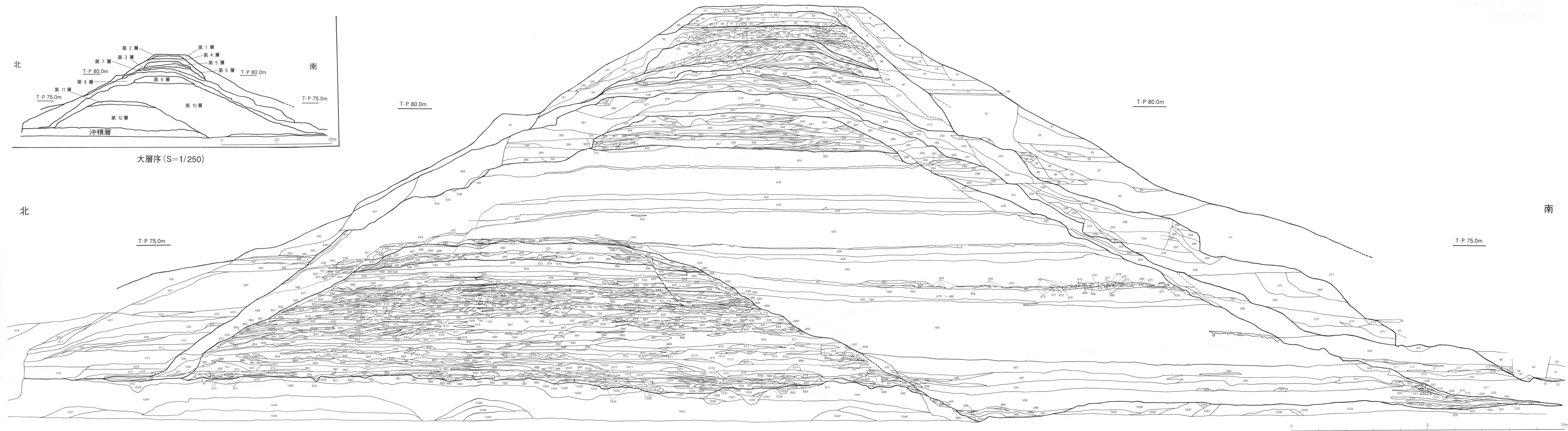
付図1 北堤断面图 (中樋地点) (S=1/50)
